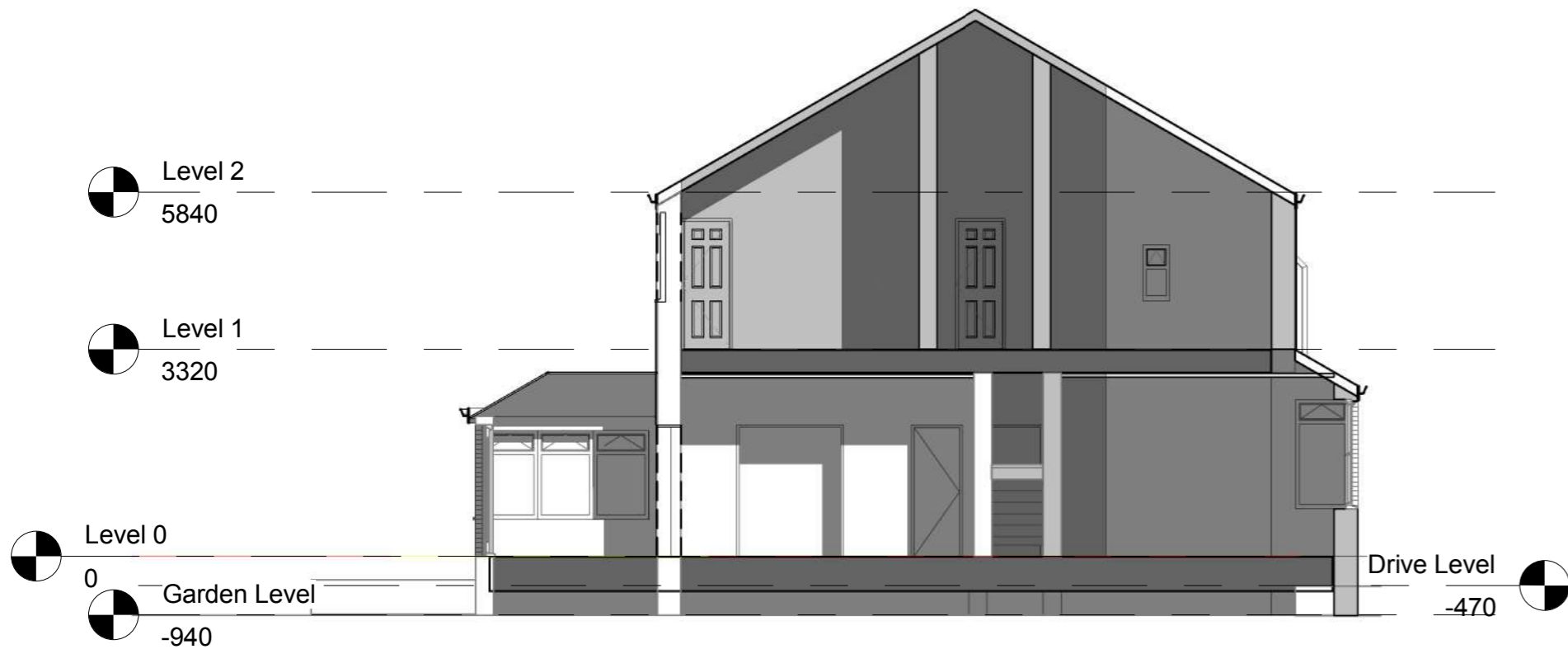
1 Long Section 1 : 100
